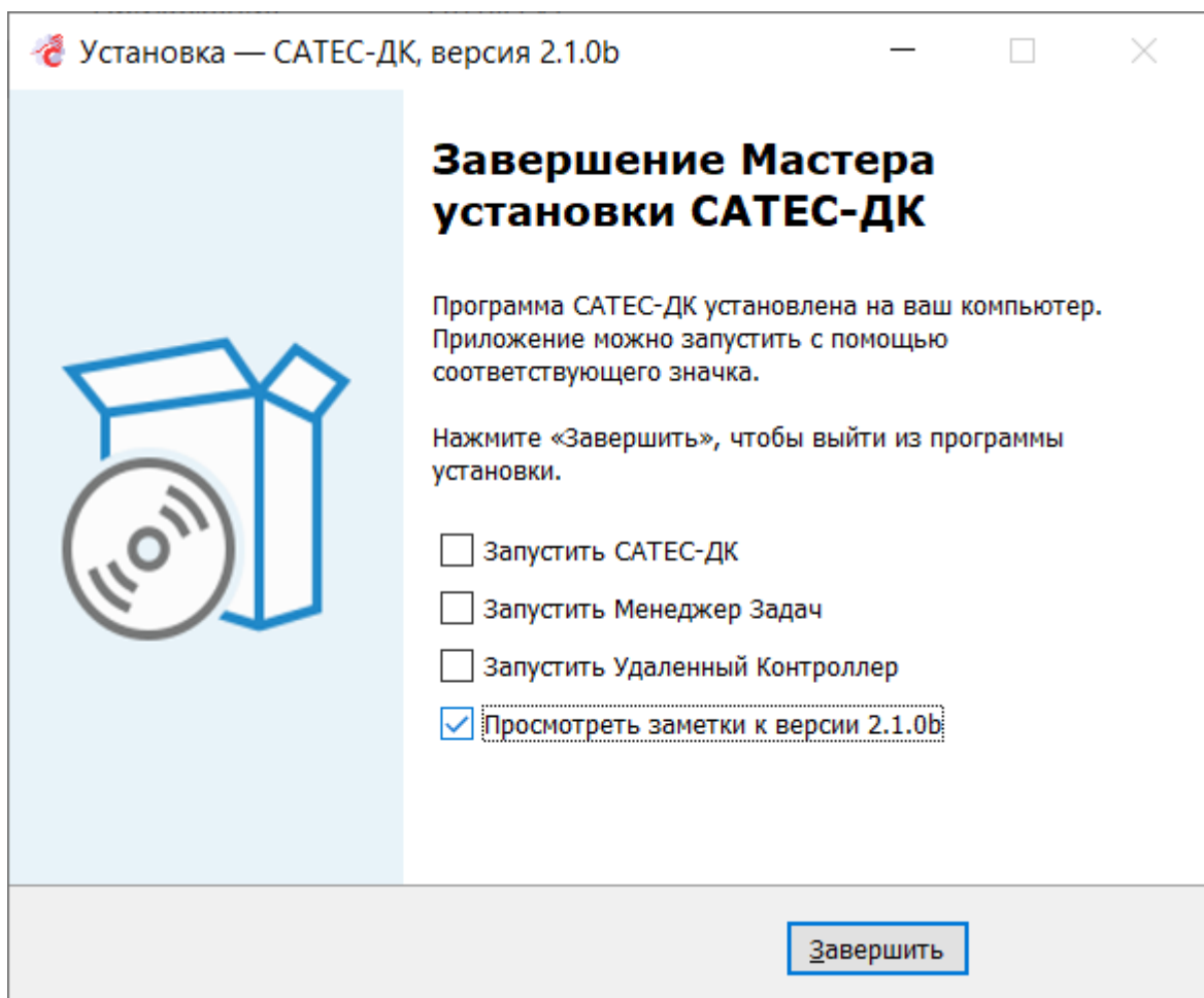
Рисунок 8 – Завершение установки
