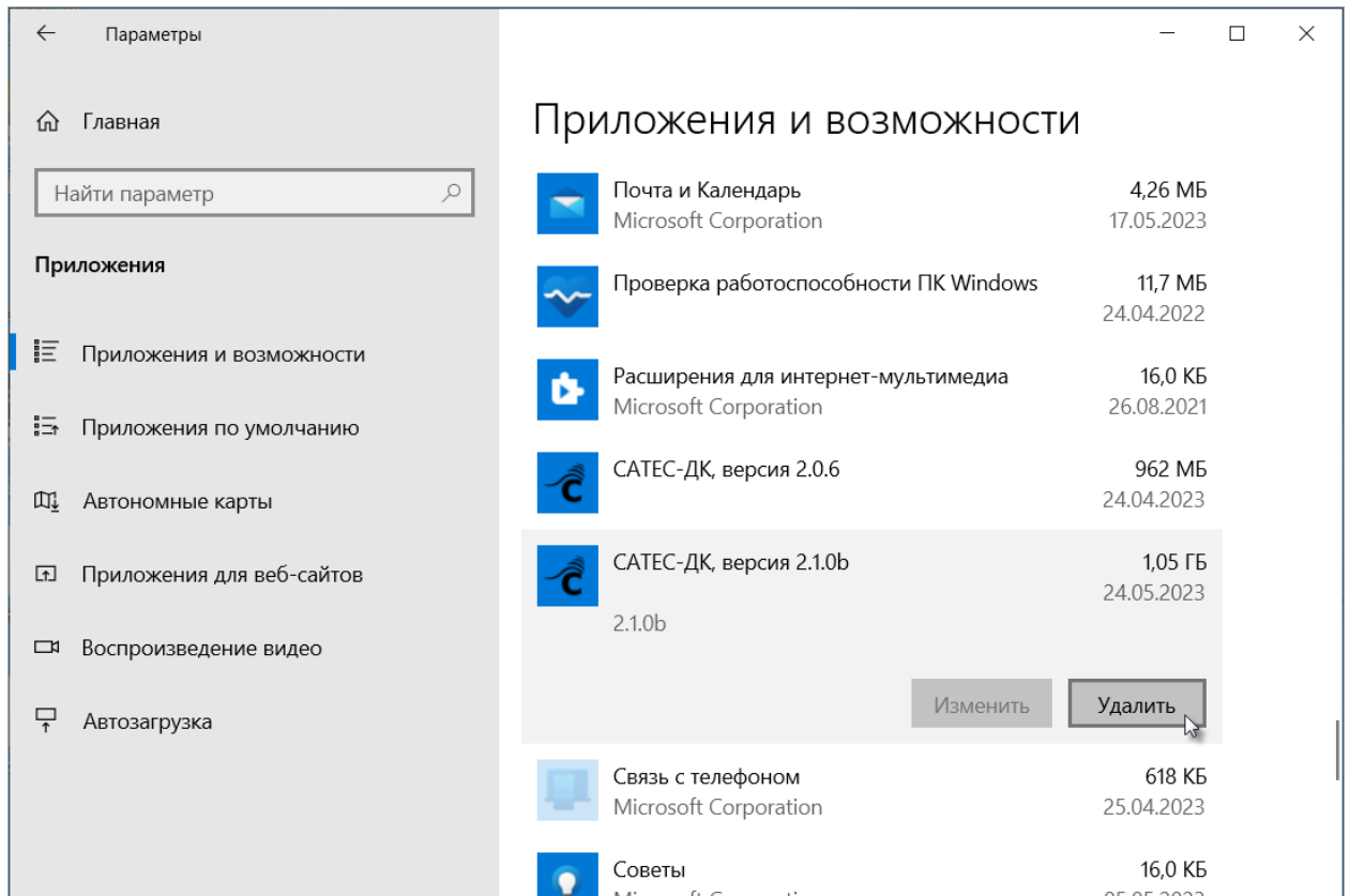
Рисунок 14 – Пункт «Удалить»
