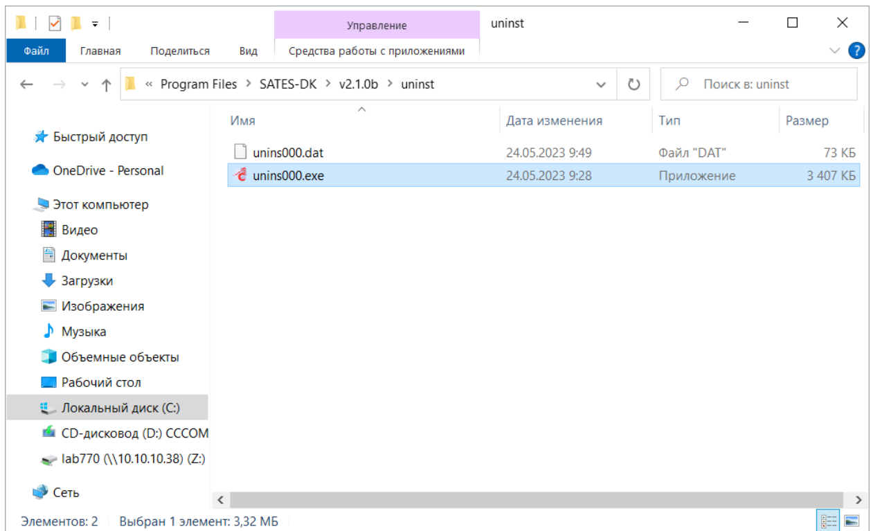
Рисунок 9 – Файл unins000.exe
